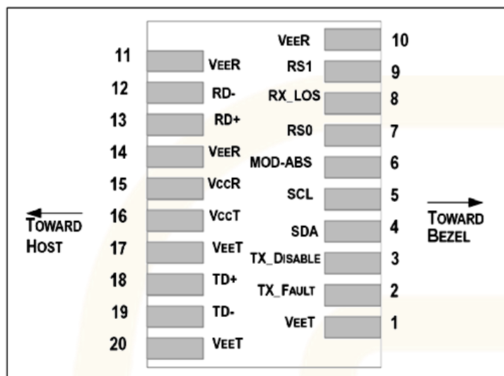
Схема основной платы с выводами
