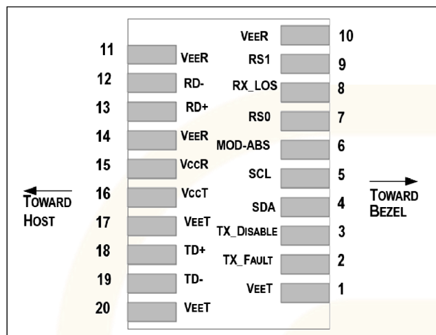
Схема основной платы с выводами
