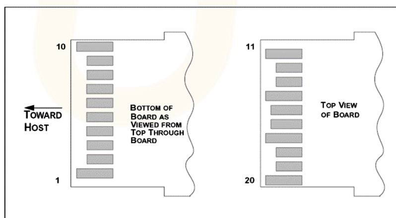
Схема основной платы с выводами
